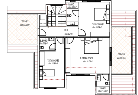
ÇATI KATI PLANI
